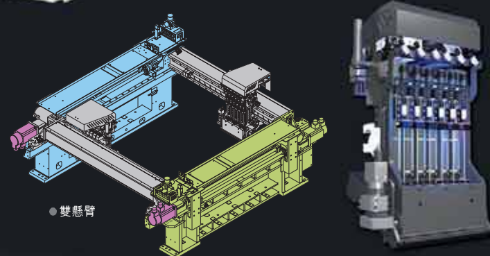
● 高速貼裝頭
