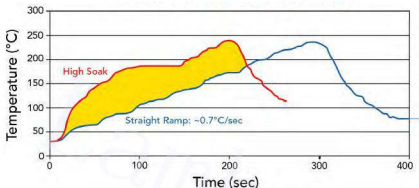
图1: CVP-390 SAC 305典型回流曲线
